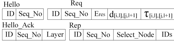
Fig. 2. Packet Formats
